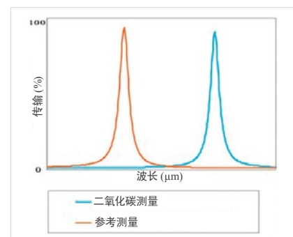
二氧化碳测量示例。参考吸收和 CO 2 吸收都是在同一光路中测量的。
