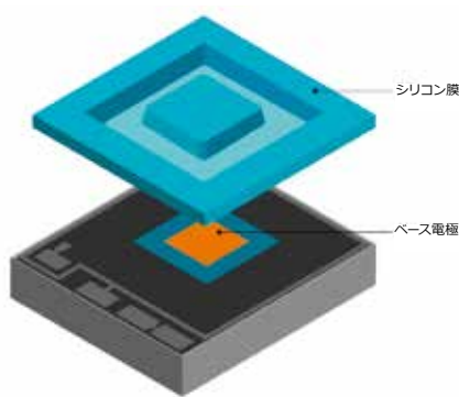
BAROCAPセンサ
