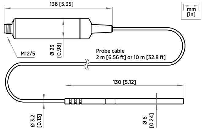
TMP1-mittapään mitat
