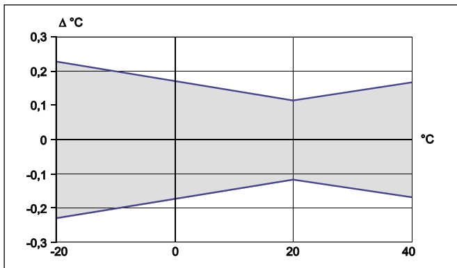
HMP155超过温度范围的测量准确度
