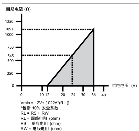
图 5 负载限制
