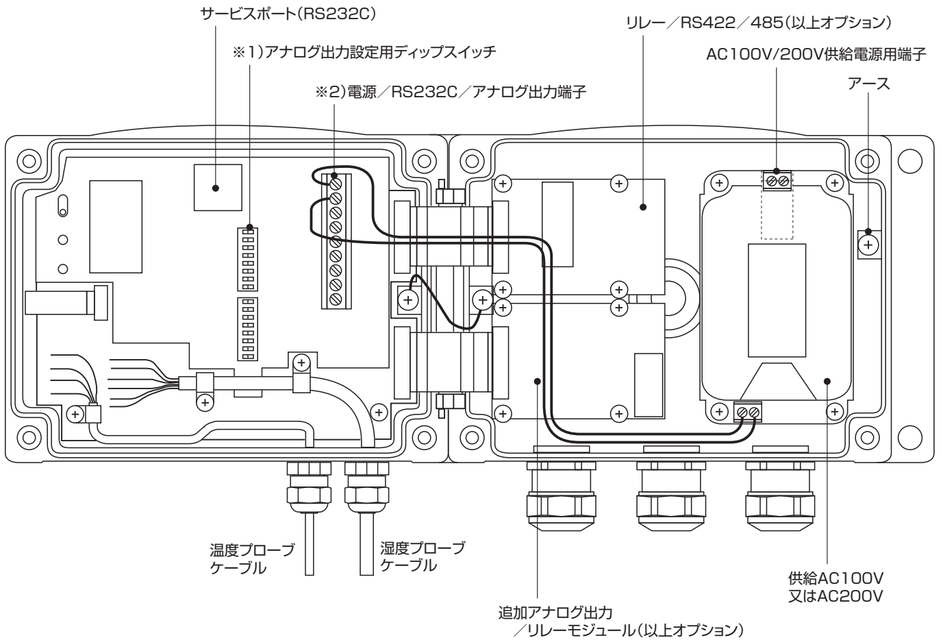
※1) アナログディップスイッチ配置図
