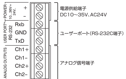
※2) 信号と電源供給の配線
