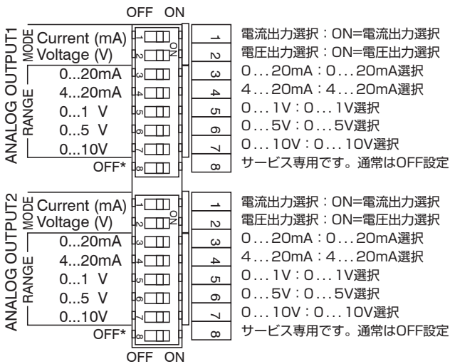
※1) アナログディップスイッチ配置図
