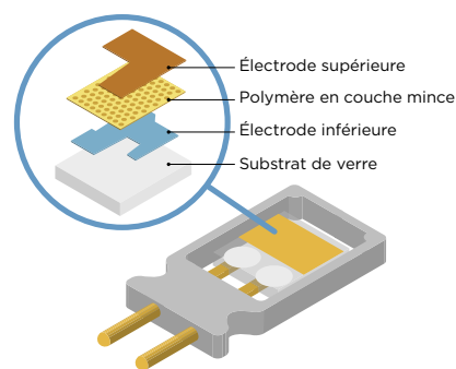
Structure du capteur HUMICAP
