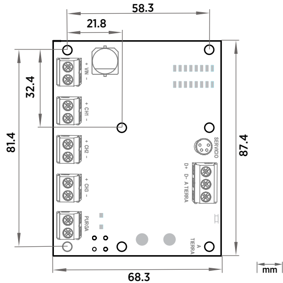
Dimensiones del panel del componente HMM170
