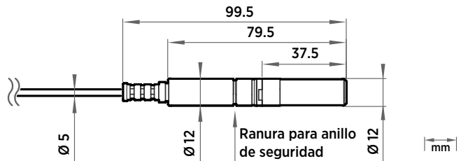
Dimensiones del cabezal de la sonda HMM170
