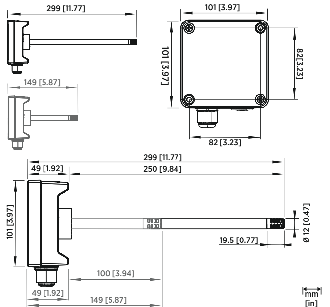
HMD60 尺寸 (长探头和短探头选选项)
