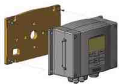
墙面安装 安装套件
