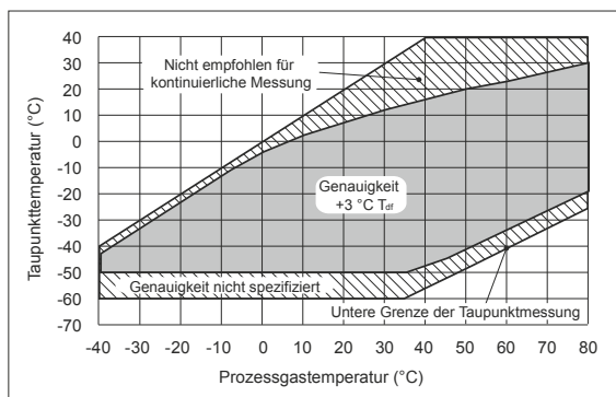
Messgenauigkeit Taupunkttemperatur
