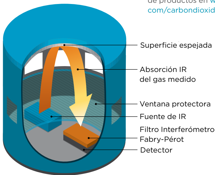
Estructura del sensor CARBOCAP®.
