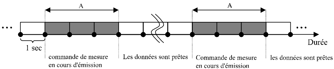
Figure 32 Méthode d'établissement de la moyenne de la mesure du vent
