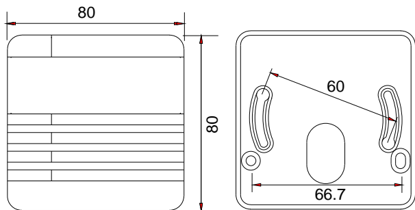
图 6 GMW22 和 GMW22D
