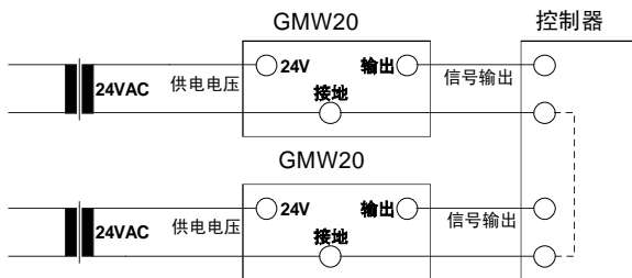
图 3 单独交流电源的连接（推荐）
