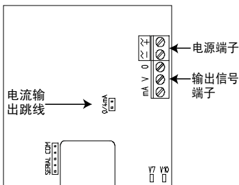
图 2 跳线和端子
