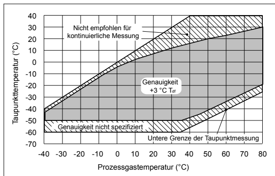
Messgenauigkeit Taupunkttemperatur
